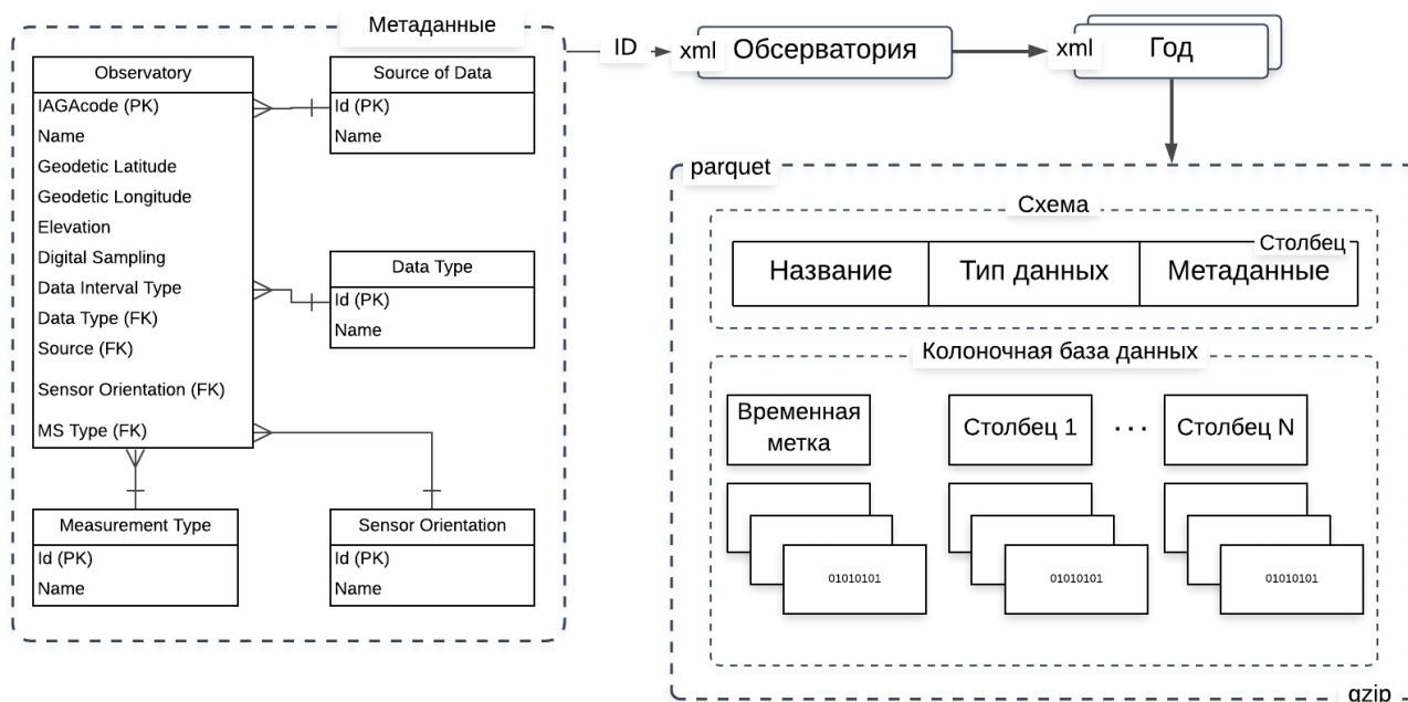
Рис. 5 Модель хранения данных в информационной системе поддержки принятия решений (на примере геомагнитной информации).
