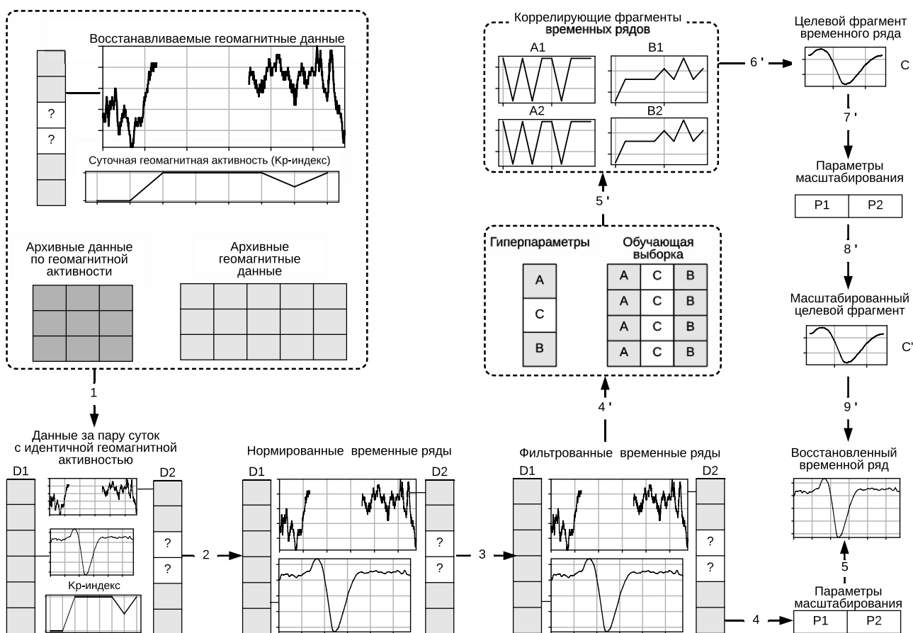
Рис. 4 Схема индуктивного метода восстановления временных рядов.
