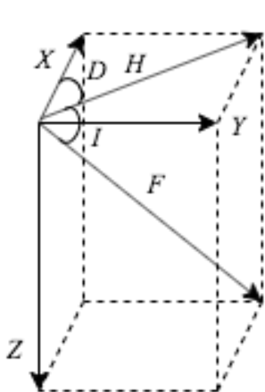
Рис. 1 Взаимосвязь компонент вектора магнитного поля Земли, выраженного геомагнитными данными.
