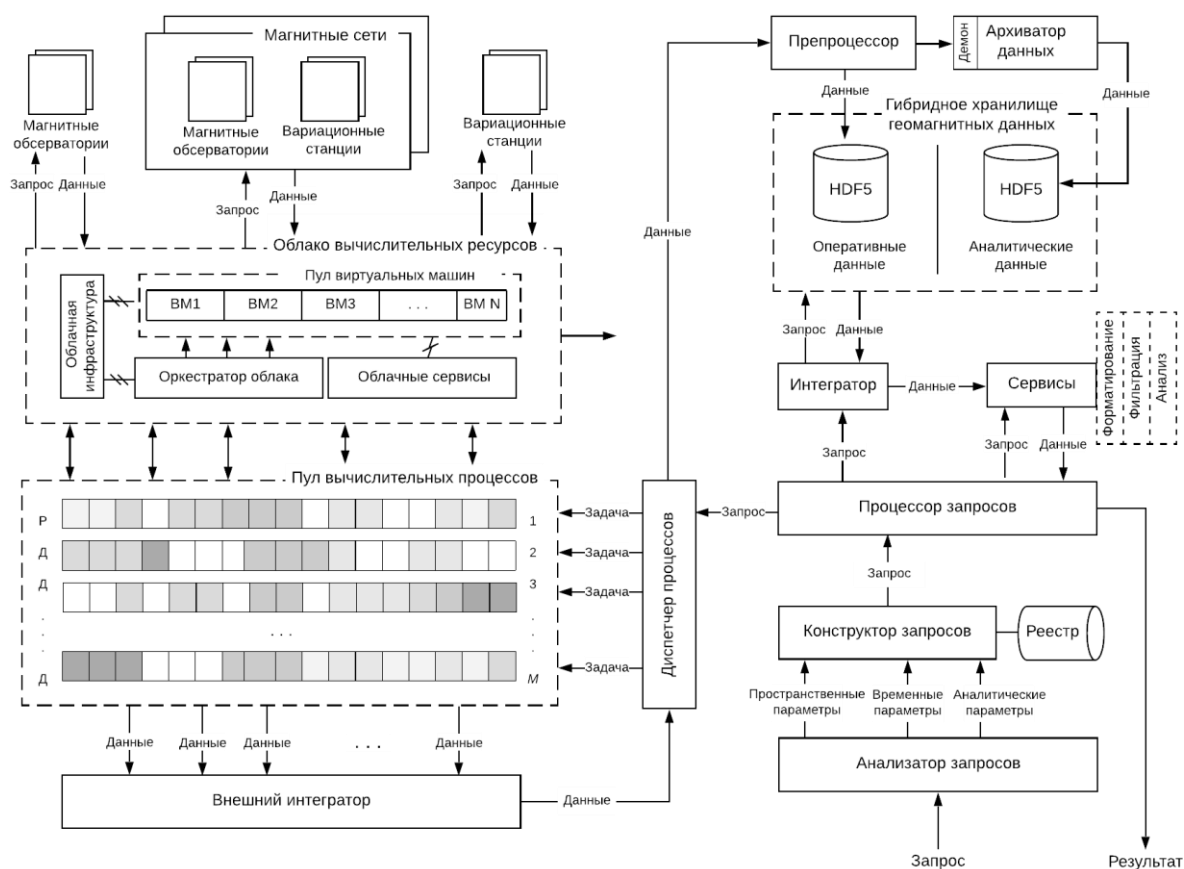
Рис. 3 Концептуальная схема единого информационного пространства на основе разнородных территориально распределенных источников (на примере геомагнитной информации).
