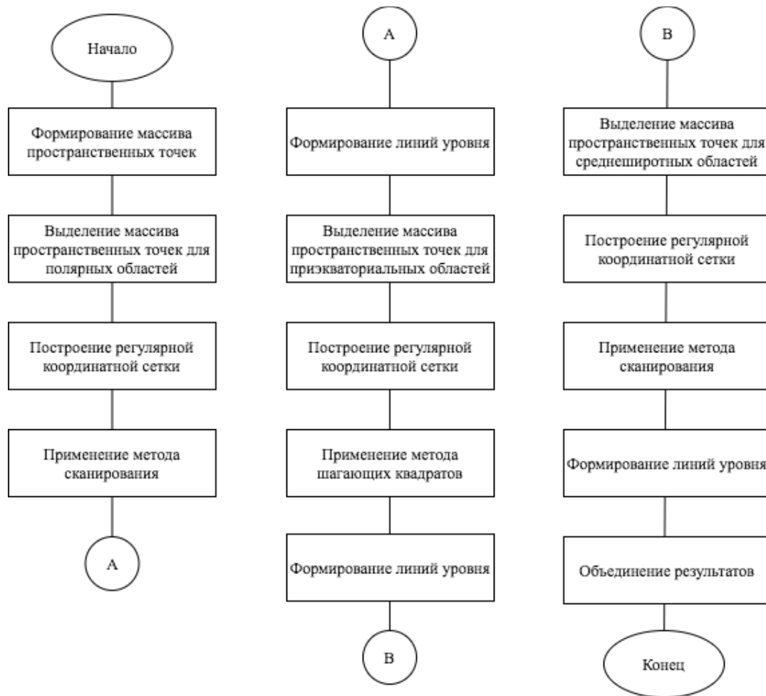
Рис. 7 Алгоритм применения гибридного метода визуализации пространственно-временного распределения геомагнитных данных.
