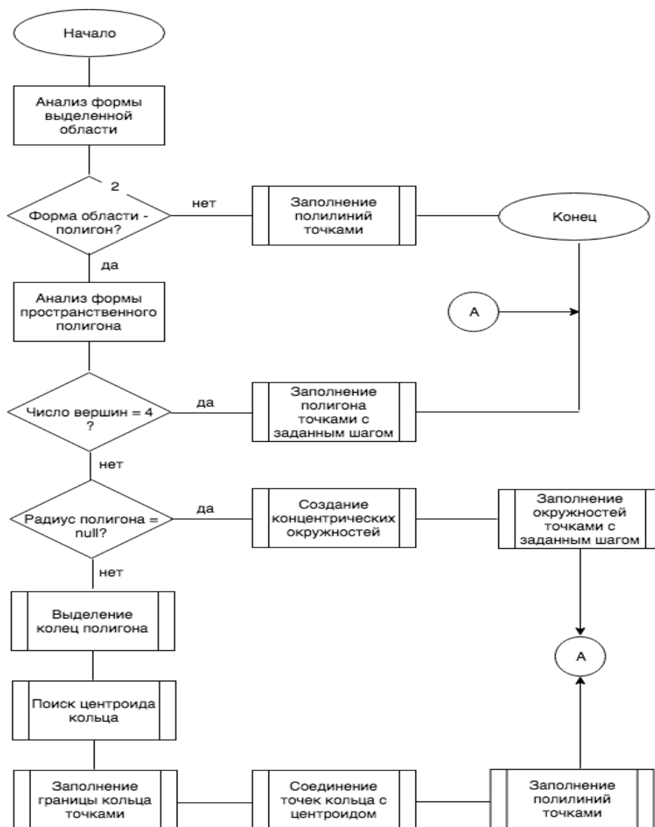
Рис. 6 Алгоритм формирования координатной сетки полигона произвольной формы.
