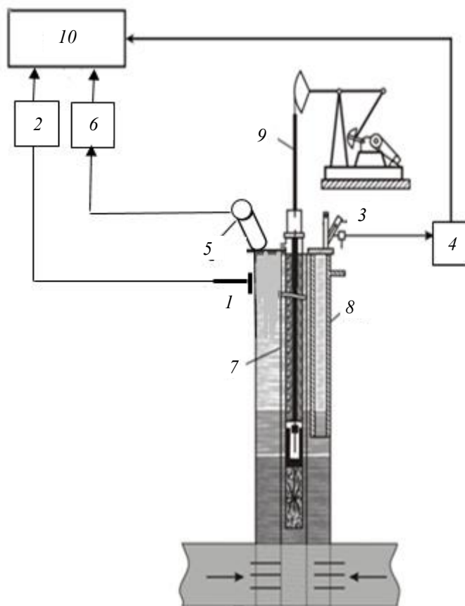
Рис. Устройство для реализации предложенного способа
